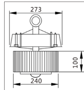
HIB1 dimensions
