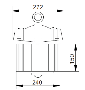
HIB2 dimensions
